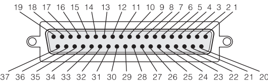
母接頭引腳圖
