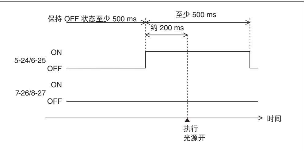
光源开的实例
