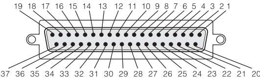
阴极接口针视图
