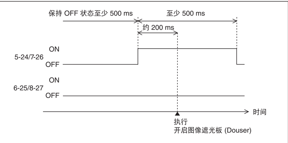
开启图像遮光板 (Douser) 的实例
