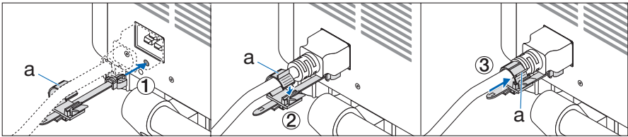
a: Abrazadera
