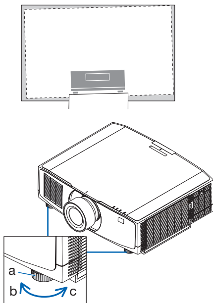
a：傾斜腳／b：上／c：下
