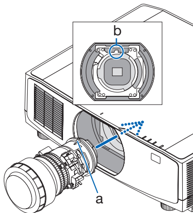
a: 突出部分 / b: 導引槽
