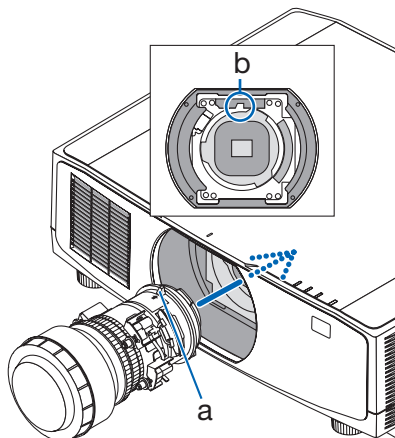
a: 돌출부 / b: 가이드 노치
