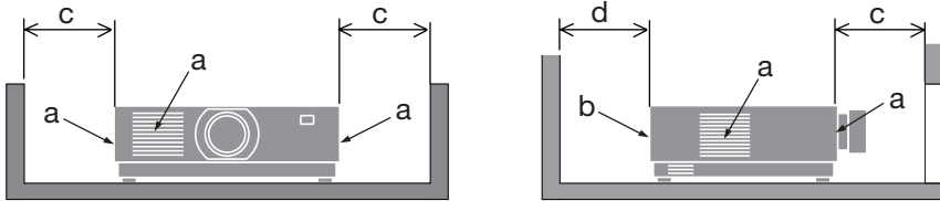
a: 흡기구 / b: 배기구 / c: 20cm / 8" 이상 / d: 30cm / 12" 이상
