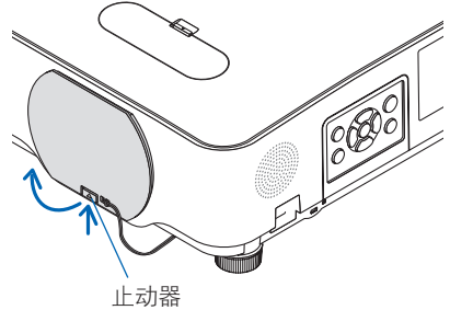
投影机单元
