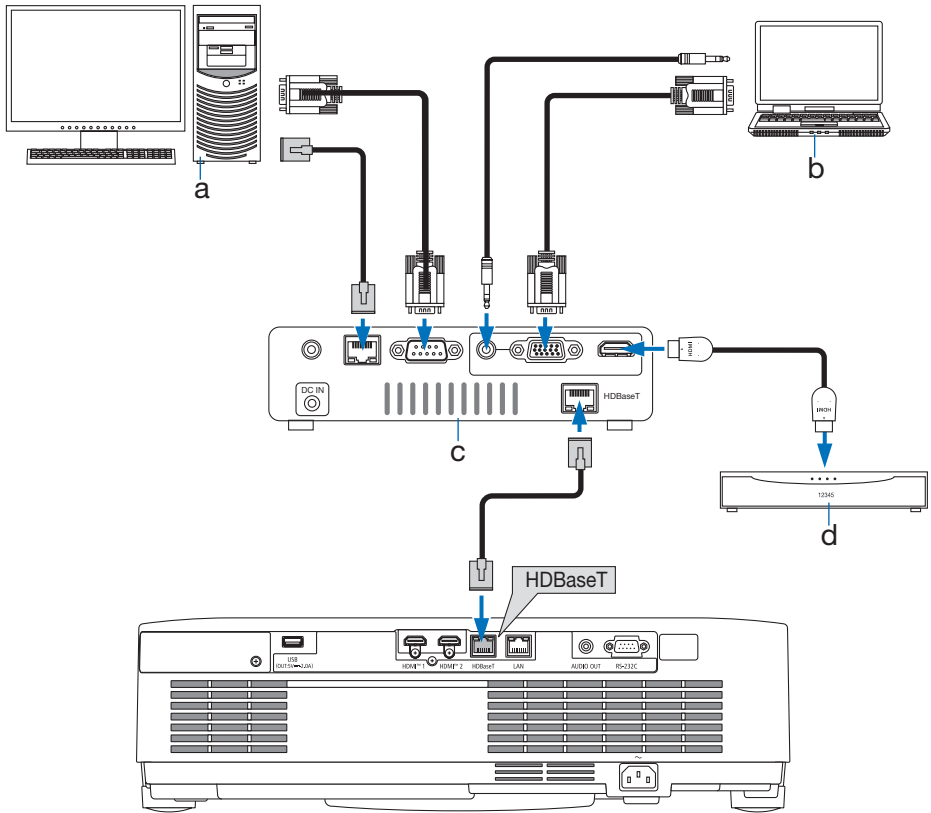
a: حاسب آلي (لأغراض التحكم) / b: حاسب آلي (لأغراض الخرج) / c: مثال لجهاز إرسال / d: جهاز فيديو بخرج HDMI
