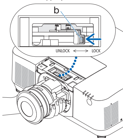
b: Μοχλός κλειδώματος φακού
