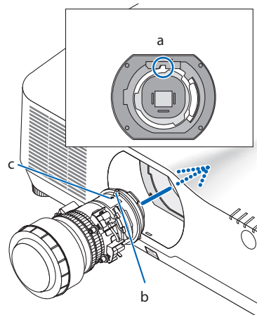
a: Ulkonema / b: Ohjauslovi / c: Nuoli
