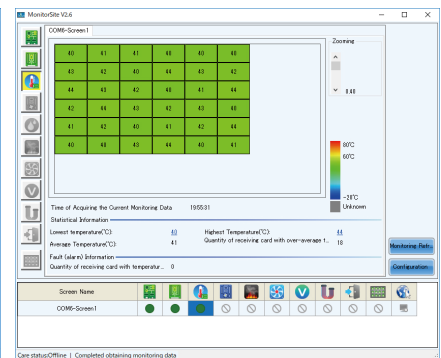
LED モジュールの温度状態表示
