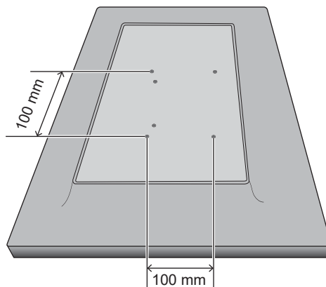
Τρύπες για βίδες για βραχίονες τοποθέτησης
